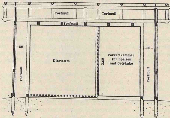
Baufüggen zu Eishütten mit Haspelmoor-Isolirung.
