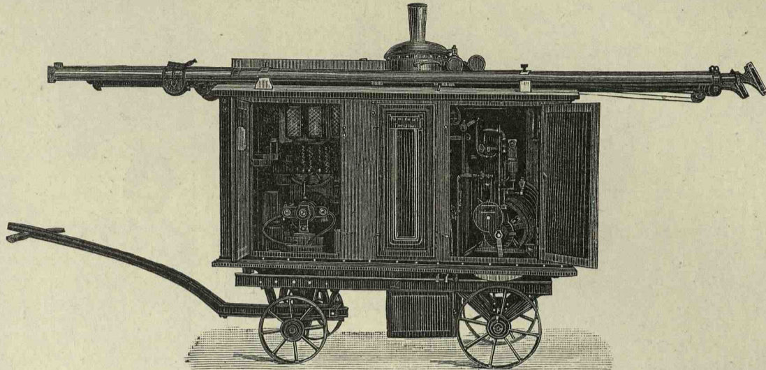
Elektrischer Beleuchtungswagen.
