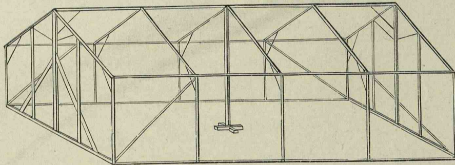
Barackenzelt System Dr. Dilms: Das Gerüst.
